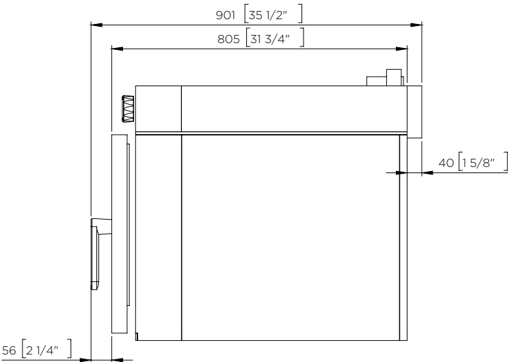
Bediening bovenop
